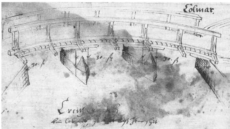
Dessin à la plume de Heinrich Schickhardt, 1596.
