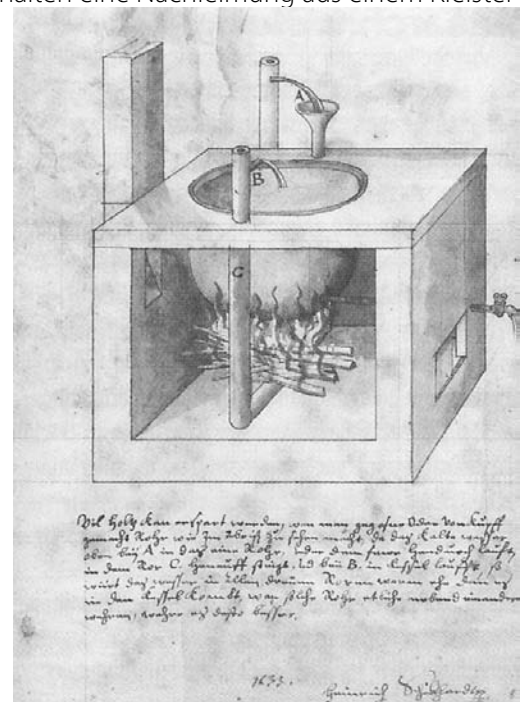
Esquisse d'un dispositif d'échauffement d'eau du bain dessinée par Heinrich Schickhardt, 1633.
